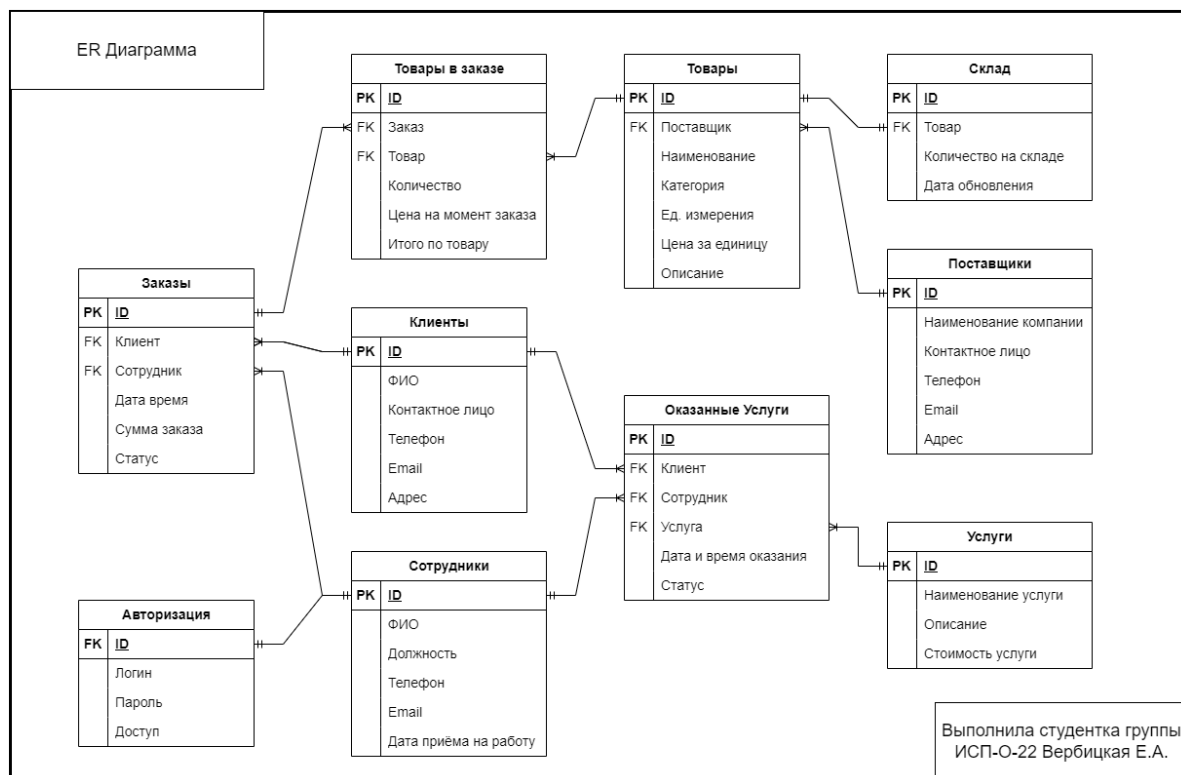
Рисунок 2.1. ER Диаграмма
