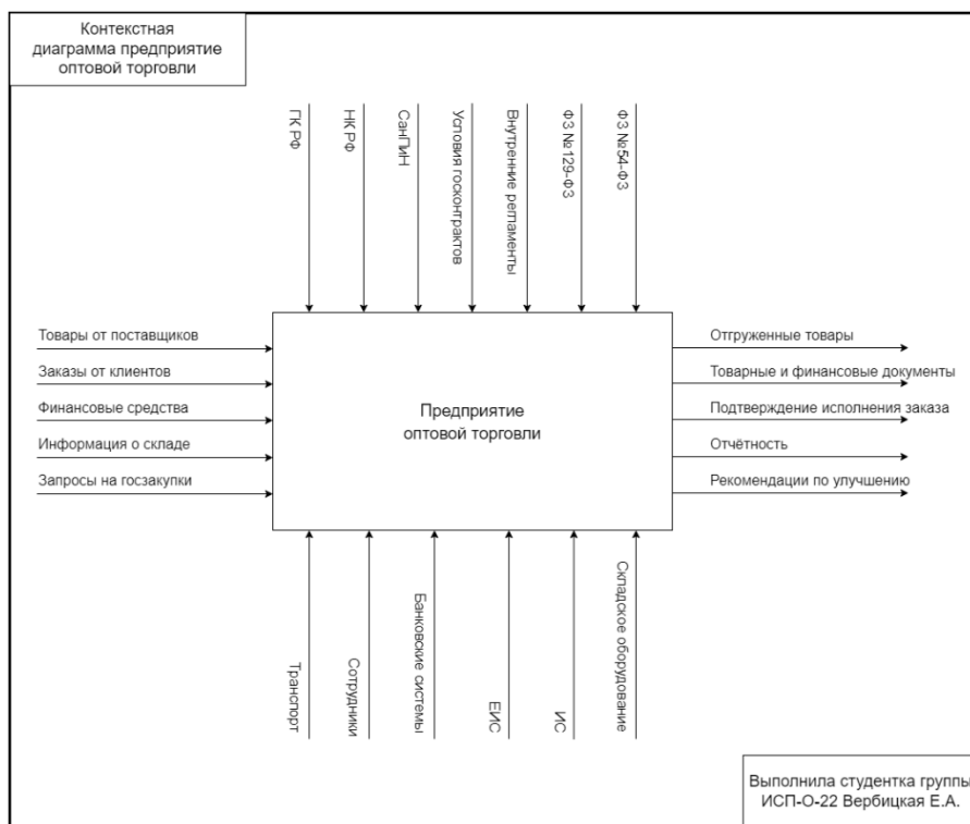
Рисунок 2.2. Контекстная диаграмма
